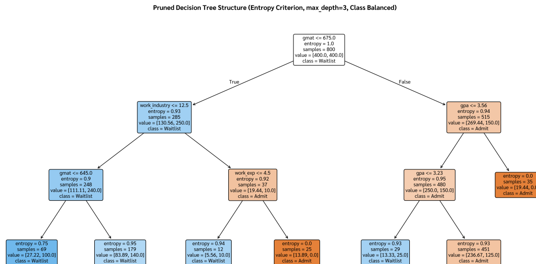
รูปที่ 2: Pruned Decision Tree Structure (Entropy Criterion, max_depth=3): แผนผังต้นไม้ตัดสินใจแสดงเงื่อนไขการตัดแบ่งในแต่ละโหนด, ค่าเอนโทรปี, จำนวนตัวอย่าง และผลลัพธ์ที่ทำนาย
